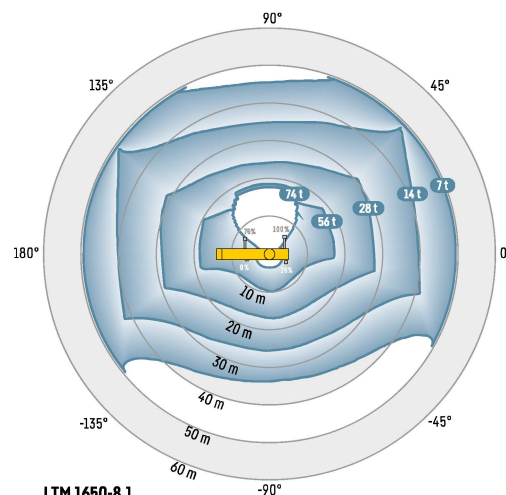
LTM 1650-8.1 54 m 100% 360° 66 t
